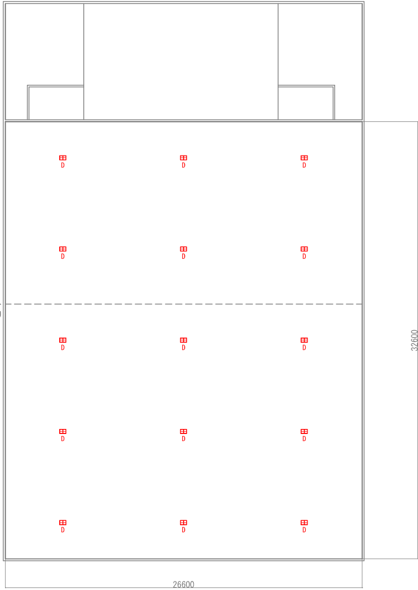
1F配灯図
