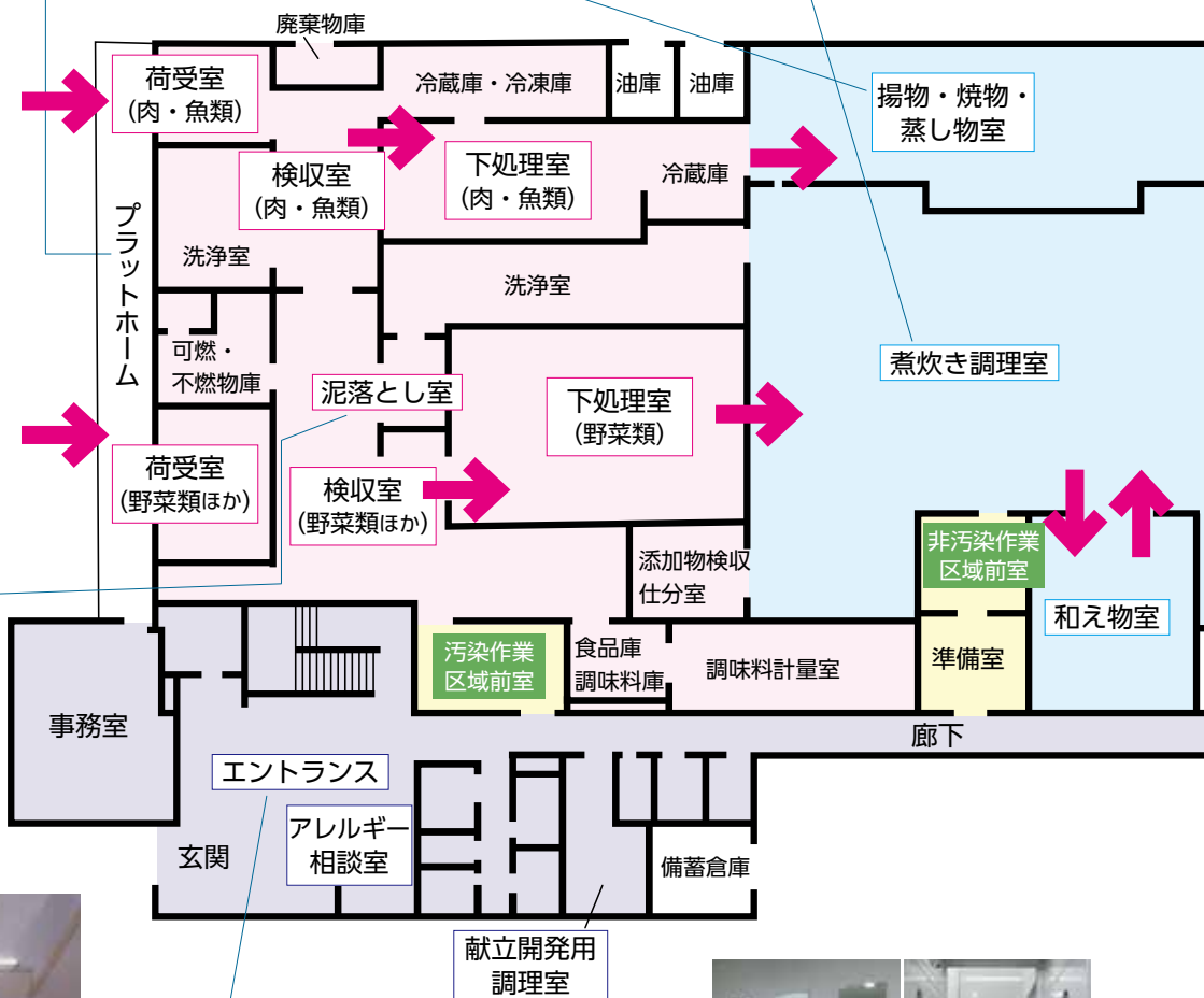
準備室・前室 汚染区域、非汚染区域ごとに設置。手洗いとエアシャワーで衛生管理を徹底しています。
