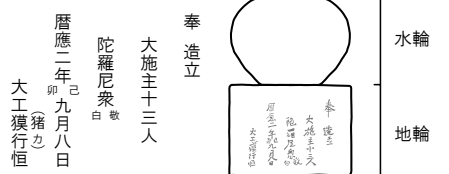
高家五輪塔復元図
